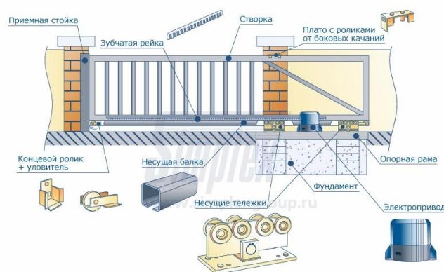
Конструкция сдвижных ворот
