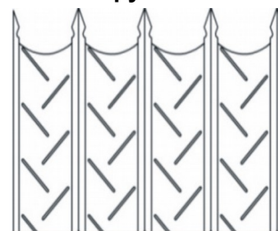
Комбинированная рубка
