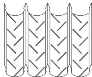
Фигурная рубка
